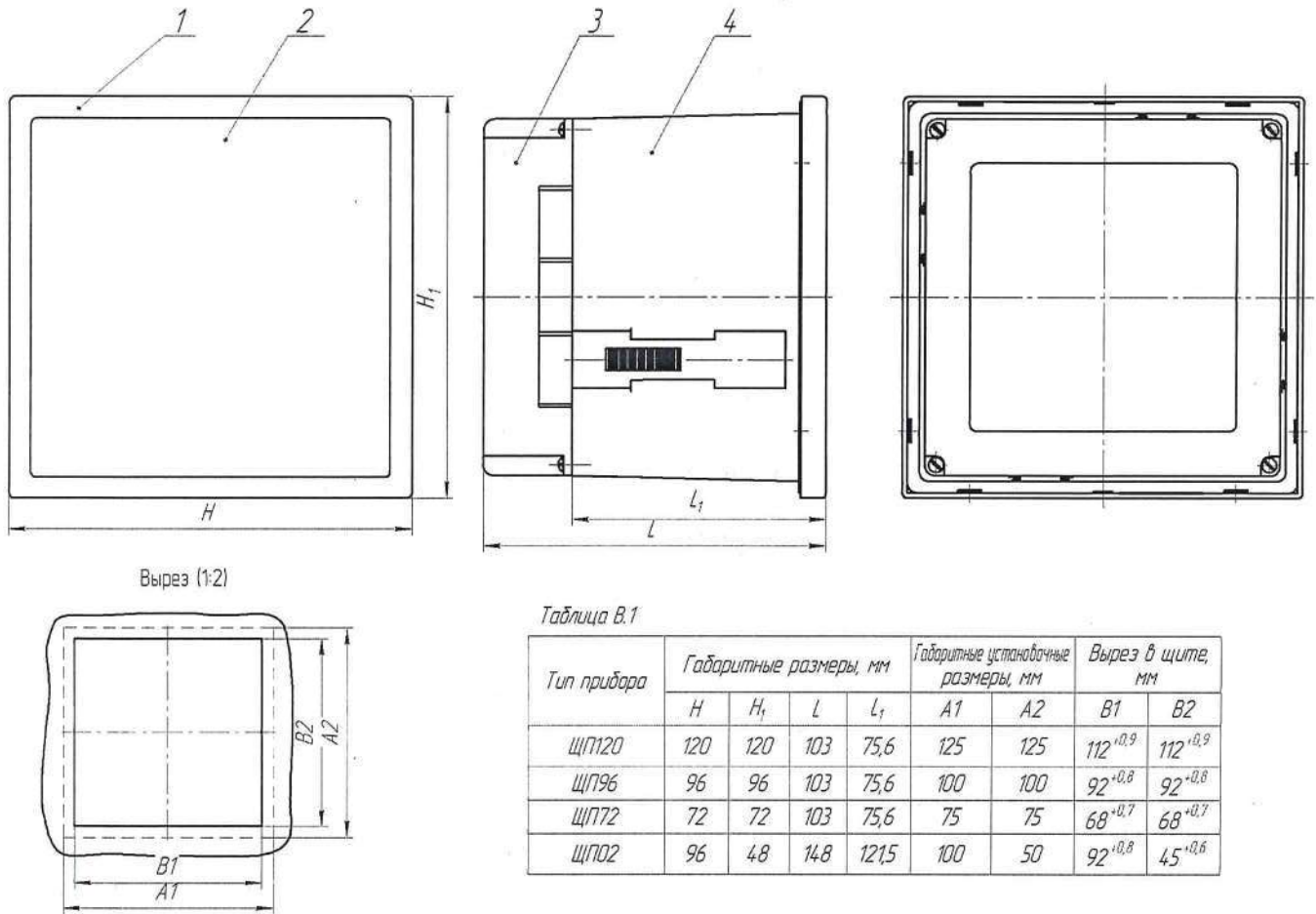
Общий вид, габаритные и установочные размеры приборов
